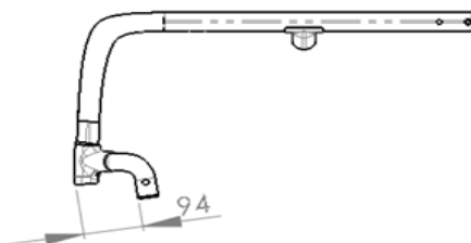
KRF010302 Ángulo más cerrado del tubo de la horquilla, y posición de la rueda retrasada
