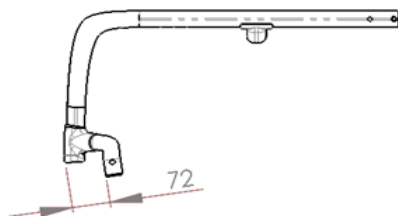
KRF010301 Ángulo standard del tubo de la horquilla, más abierto, y posición de la rueda adelantada
